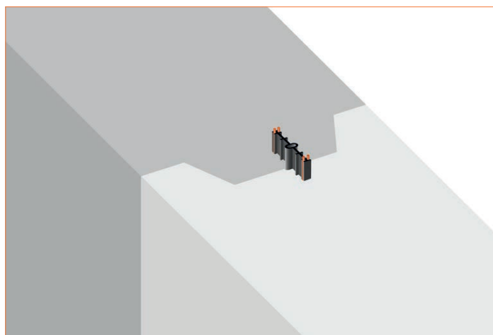
6. Giunto impermeabilizzato perpendicolarmente dal Nastro Waterstop DRYset.
